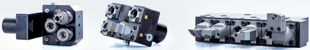
Feststehende und angetriebene Werkzeughalter
